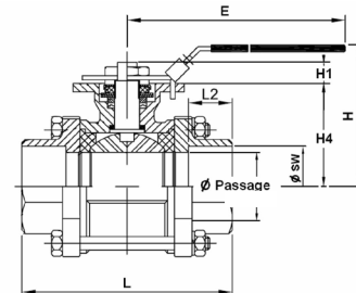
Modèle à souder : SW
