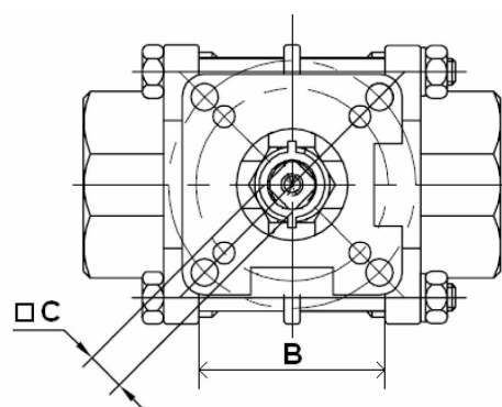
Modèle à souder : SW
