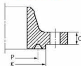
Face usinée pour joint annulaire Ring-joint face
