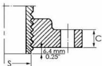
Emboitement mâle étroit Small male face
