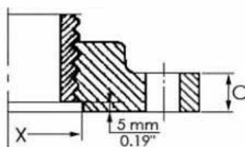
Emboitement femelle étroit Small female face
